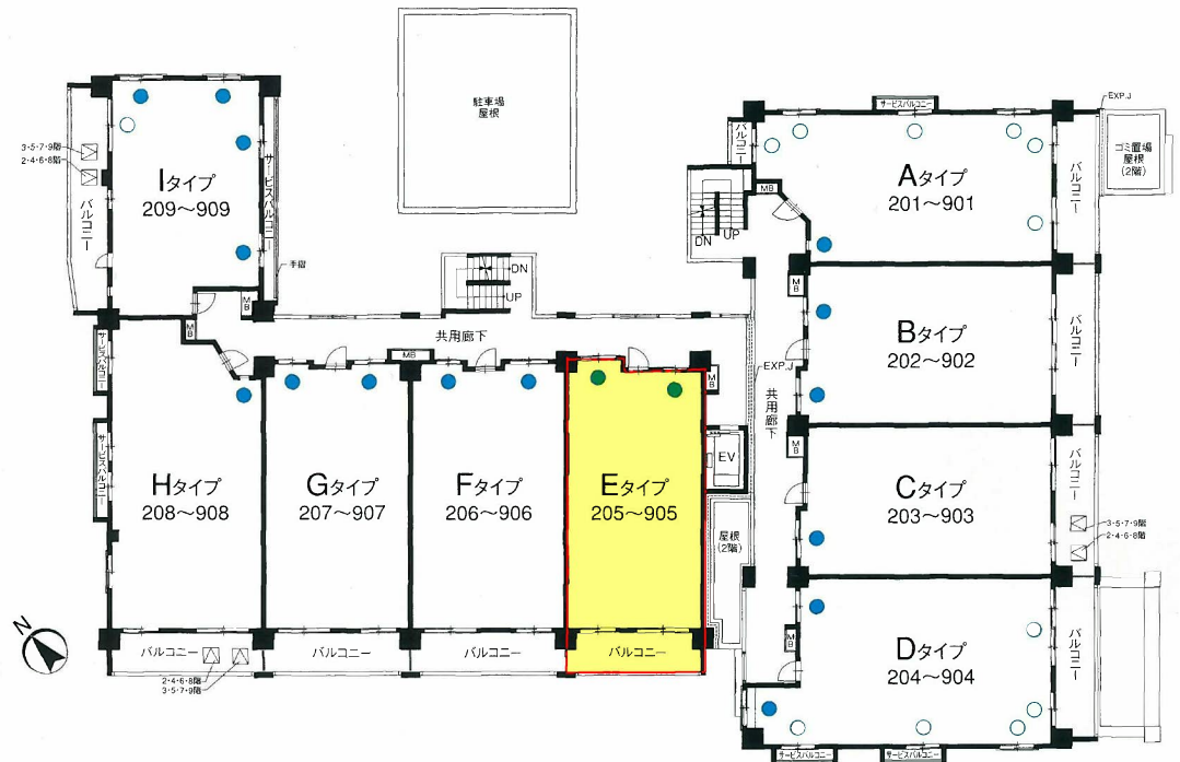
2~9階平面図
